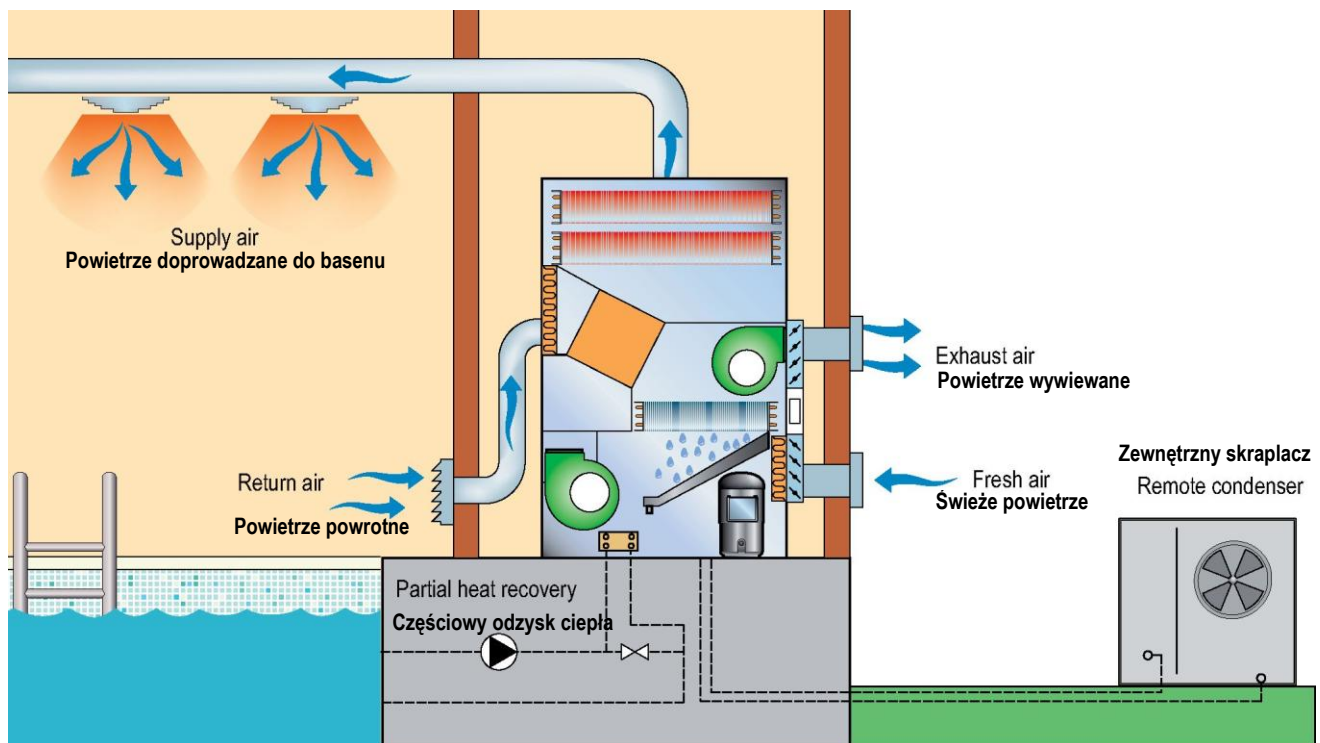
SCHEMAT INSTALACJI Z UTAZ
